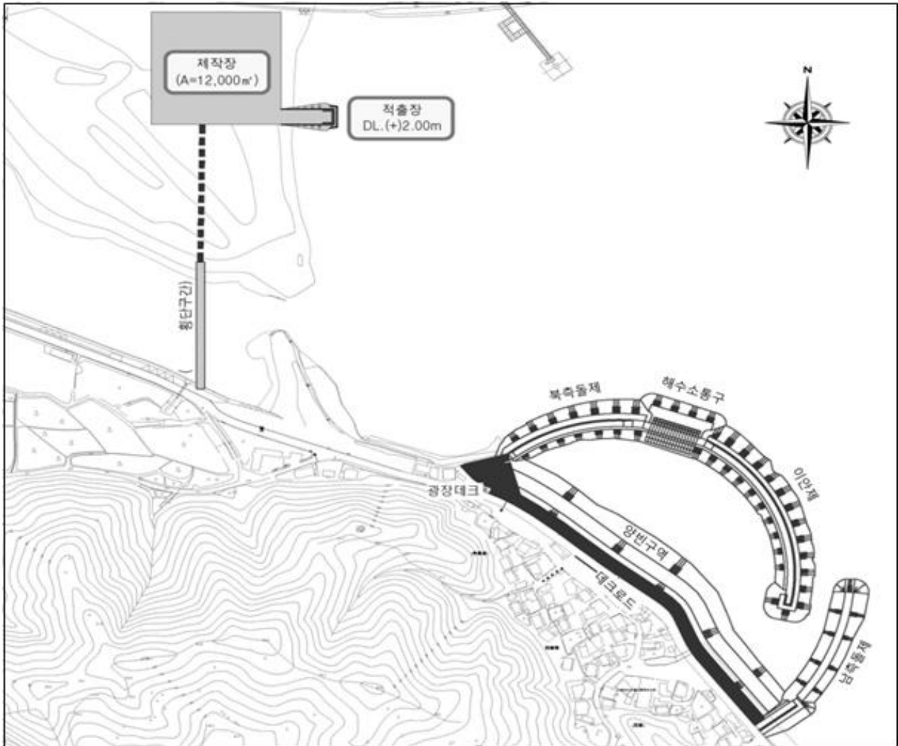
【그림 1】 ○○ ■■■연안 복원공사 공사계획도
